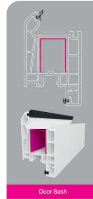
Door Sash
